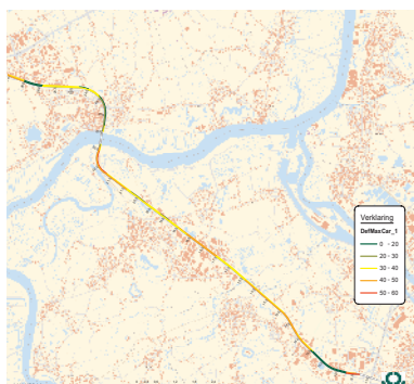
Karakteristieke maximale deflectie op een deel van de N16
